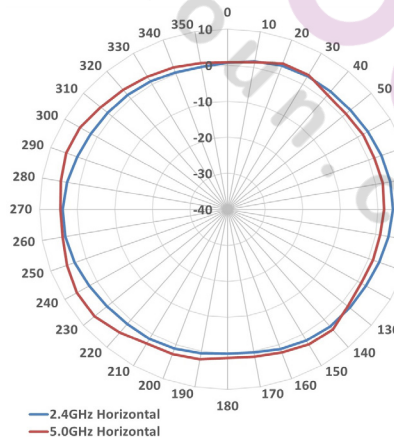
H-Plane Pattern
