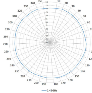
H-Plane Pattern Radio1 Horizontal
